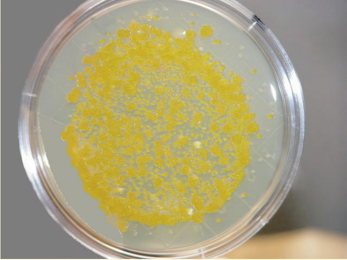
PCA
